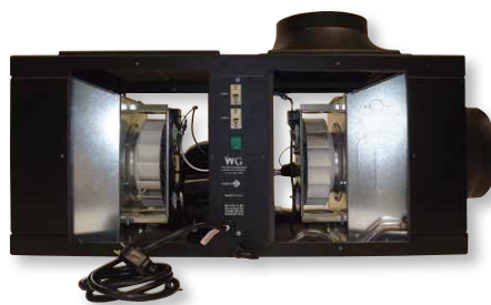
Seitenansicht mit Standard-Manschetten für den Eingangs- und Rückkanal (Abdeckungen entfernt)
